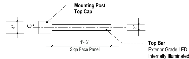
6 TOP VIEW - SIDE B SCALE: 1" = 1'-0"
