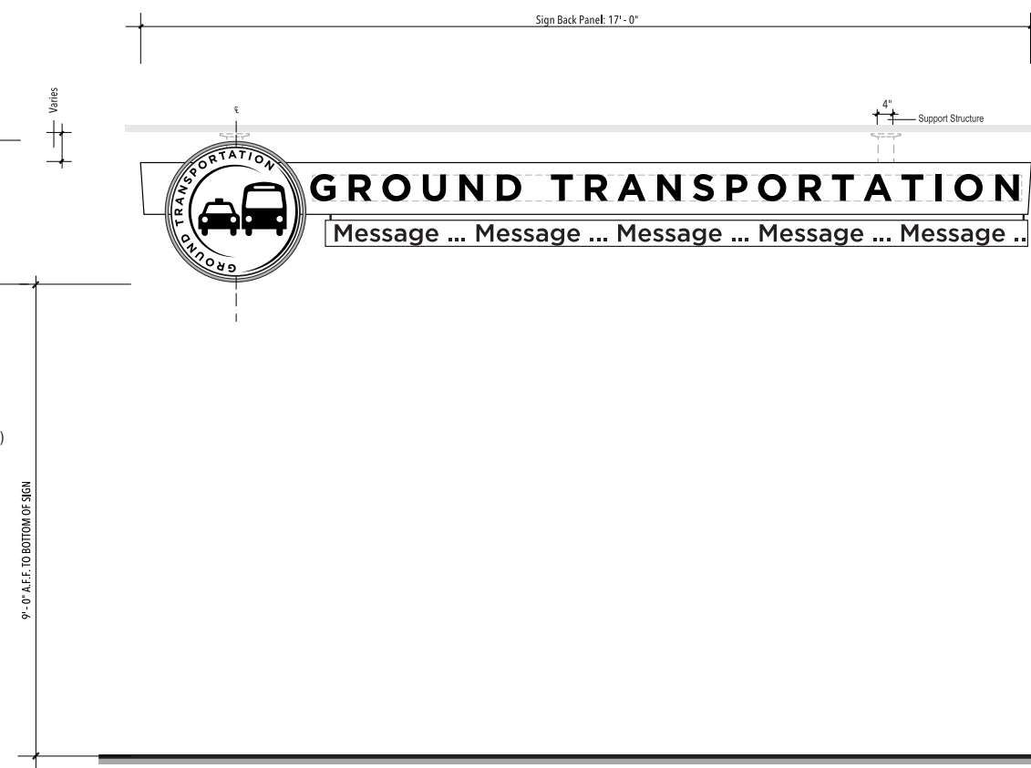
5 ELEVATION SCALE: 1/2" = 1'-0"
