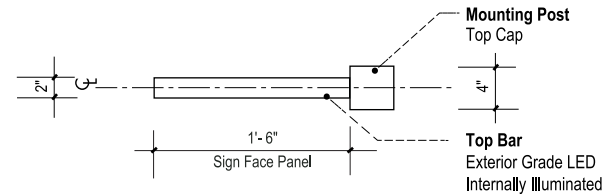
1 TOP VIEW - SIDE A SCALE: 1" = 1'-0"
