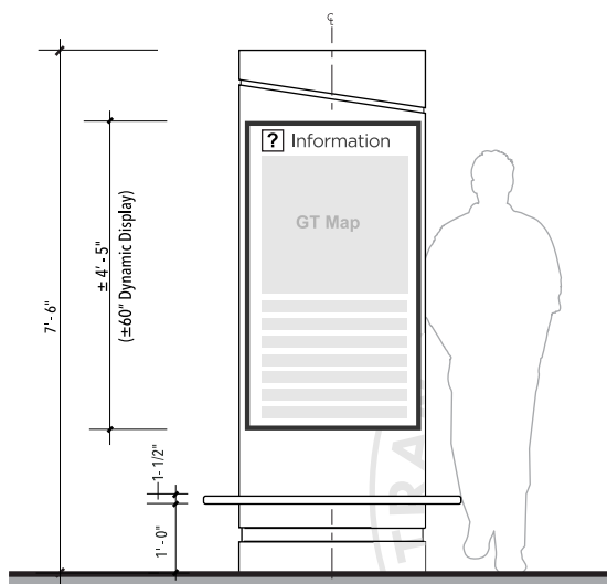
5 FACE LAYOUT - SIDE A SCALE: 1/2" = 1'-0"
