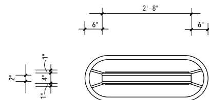
1 TOP VIEW SCALE: 1/2" = 1'-0"
