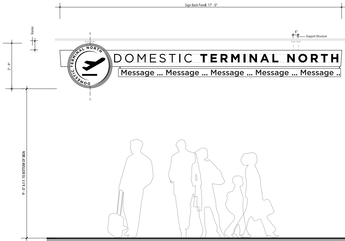
5 ELEVATION SCALE: 1/2" = 1'-0"
