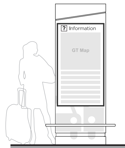
5 FACE LAYOUT - SIDE B SCALE: 1/2" = 1'-0"
