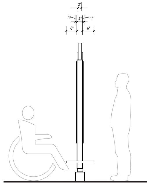
6 SIDE VIEW SCALE: 1/2" = 1'-0"
