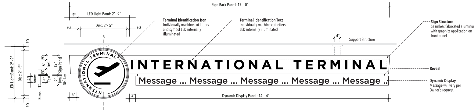
1 FACE LAYOUT - SIDE A SCALE: 1/2" = 1'-0"
